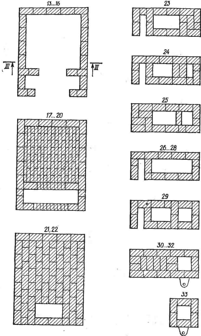
Рис. 34. Русская печь:
