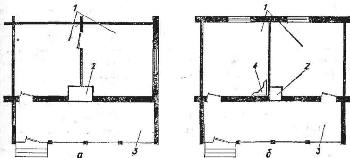
Рис. 17. Размещение печи ( а ), а также печи и камня ( б ) в зданиях дачного или садового типа:
