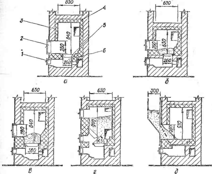
Рис. 12. Конструкции топливников:
