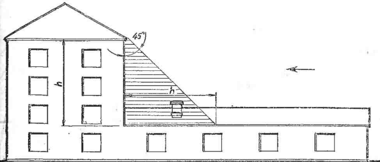
Рис. 47. Размещение дымовой трубы в зоне ветрового подпора.
