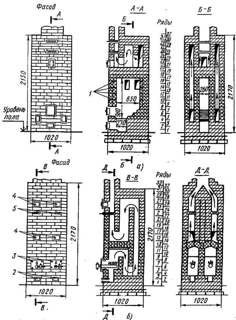
Рис. 52. Перевод большой отопительной печи с твердого топлива на газ с разделением ее на две печи с самостоятельными топливниками в том же массиве:
