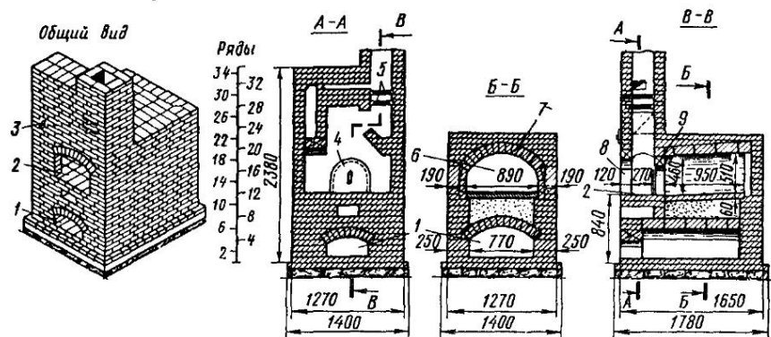
Рис. 30. Обыкновенная русская печь:
