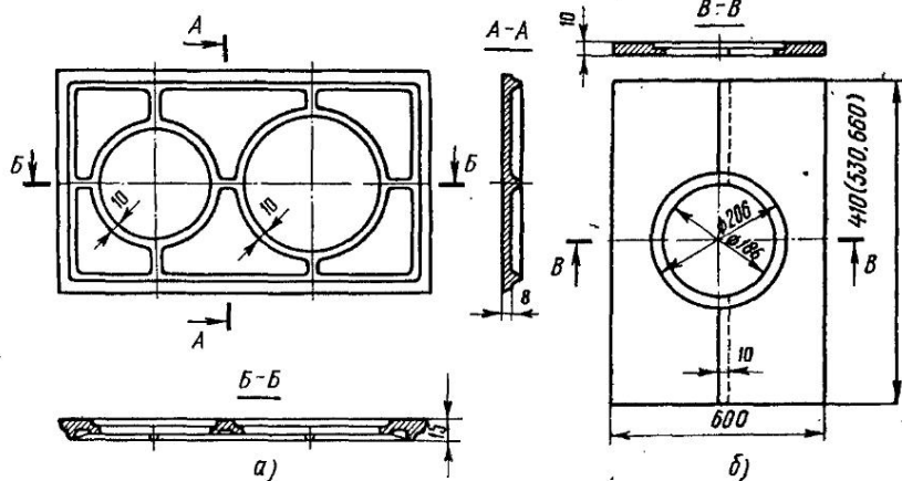
Рис. 63. Чугунные плиты: а — цельная, б — составная
