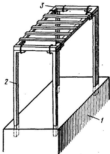
Рис. 77. Основание под печь верхнего этажа в виде металлической рамы: 1 — фундамент, 2 — стойки, 3 — металлическая рама
