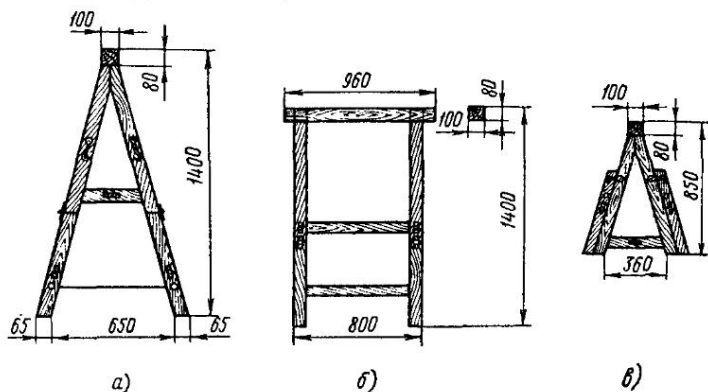
Рис. 69. Усовершенствованные подмости:
