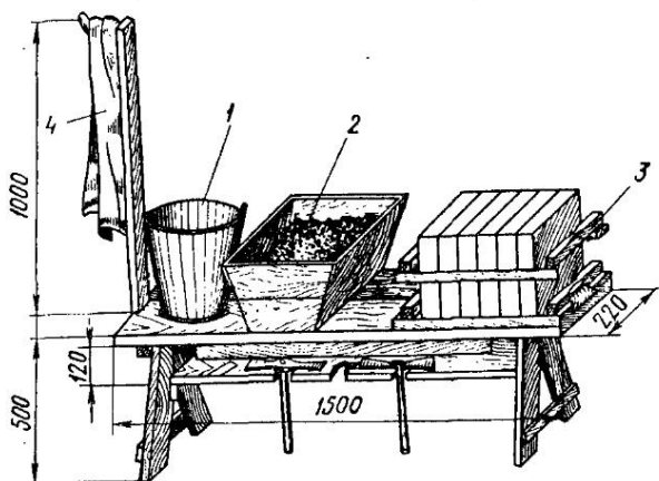
Рис. 70. Скамья для материалов и инструмента:
