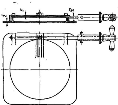
Рис. 62. Поворотная заслонка
