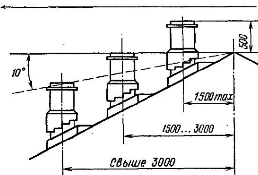
Рис. 13. Расположение дымовых труб над крышей
