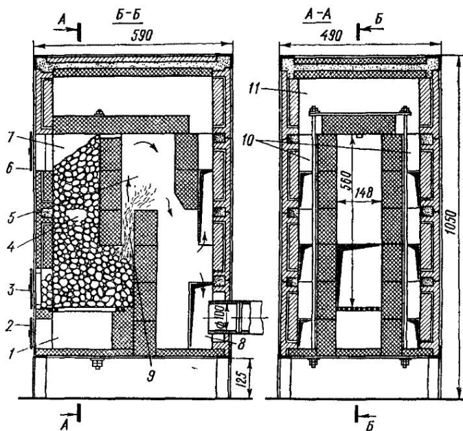
Рис. 25. Печь АКХ-9 длительного горения на твердом топливе: 1 — зольник, 2 — поддувальная дверка, 3 — топочная дверка 4 — топливник с колосниковой решеткой, 5 — промежуточная кла- мера, 6 — дверка для загрузки топлива, 7 — шахта, 8 — коллектор, 9 — средний канал, 10 — боковые каналы, 11 — выход двух каналов над перекрытием камеры
