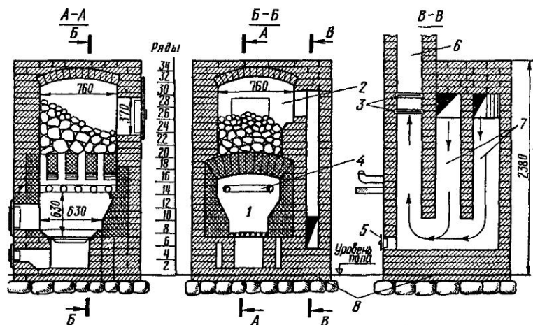
Рис. 41. Банная печь-каменка:
