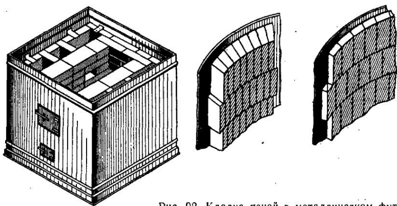
Рис. 92. Кладка печей в металлическом футляре
