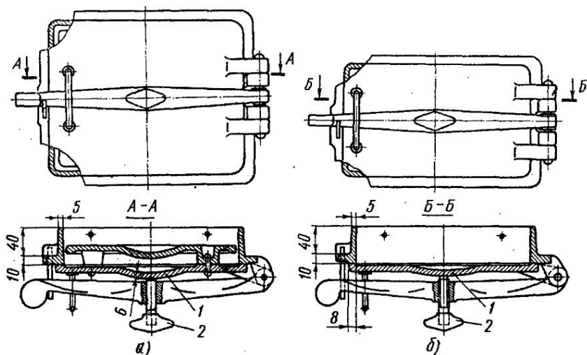
Рис. 58. Герметические дверка (а) и полудверка (б):
