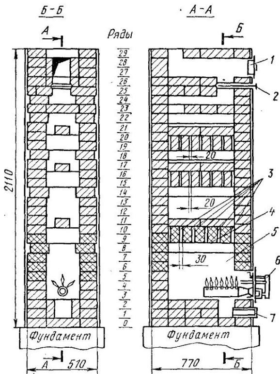
Рис. 50. Газовая отопительная печь АКХ-14:
