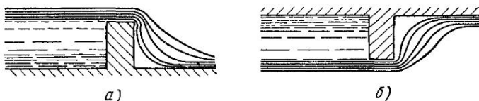
Рис. 2. Обтекание порога в канале: а — водой, б — газом
