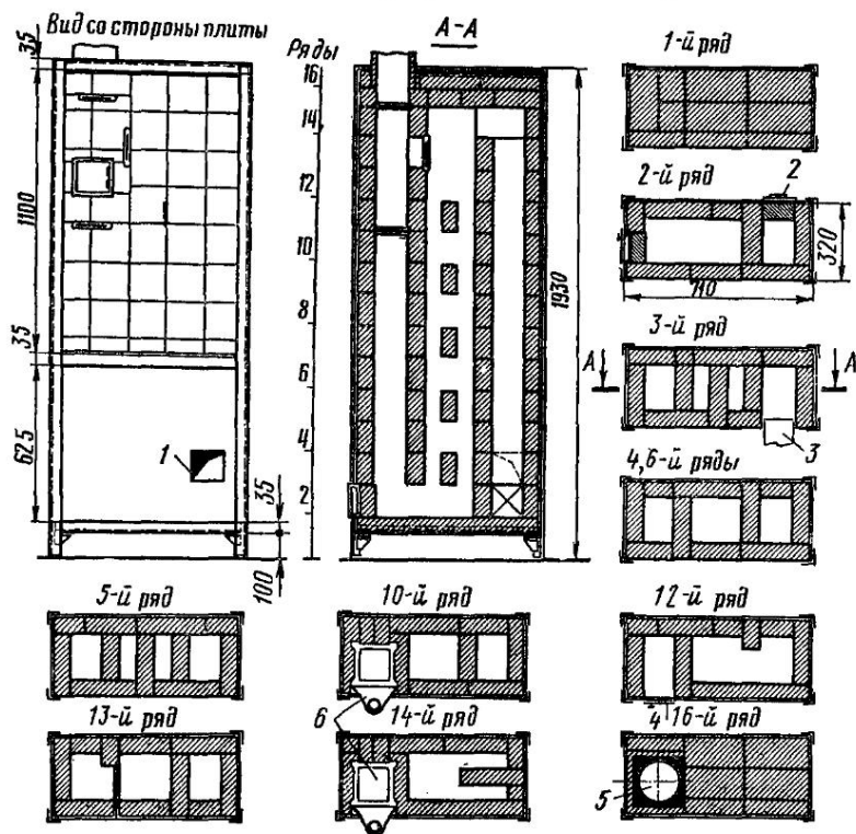
Рис. 35. Отопительный щиток кирпичный облегченной конструкции ОЩК-1: 1 — место присоединения плиты к щитку, 2 — чистка, 3 — стальной патрубок, 4 — самоварник, 5 — асбестоцементная труба, 6 — задвижки
