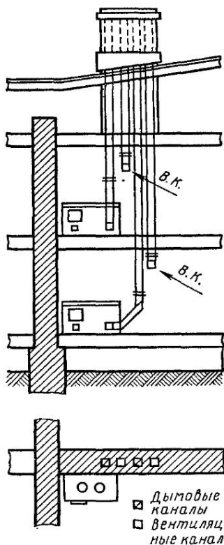
Рис 14. Размещение дымовых каналов в стене двухэтажного здания
