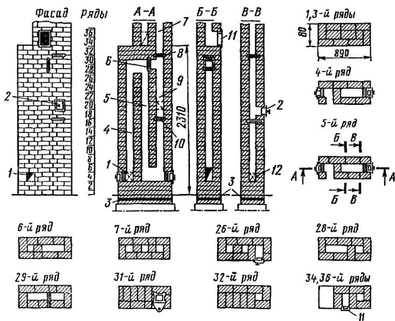
Рис. 34. Отопительный щиток толстостенный ЩИТ-1:
