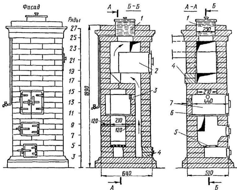
Рис 37 Отопительно-варочная печь конструкции В. А. Цотанова. 1 — водогрейная коробка, 2 — духовой шкаф, 3 — вытяжной канал, 4 — чистка, 5 — ко- лосниковая решетка, 6 — чугунная плита, 7 — варочная камера
