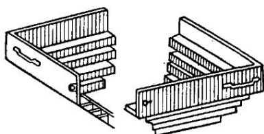
Рис. 71. Инвентарный шаблон для устройства горизонтальных разделок у трубы
