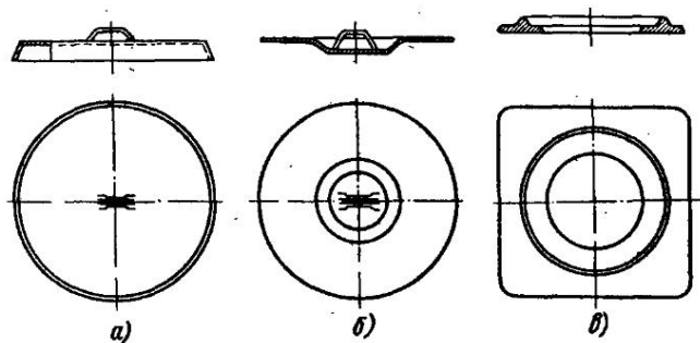
Рис. 60. Чугунная вьюшка: а — крышка, б — блинок, в — рамка
