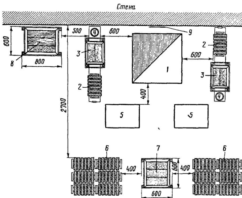
Рис. 104. Схема организации рабочего места при кладке печи у стены: 1 — печь, 2 — рамки с кирпичом, 3 — расходные ящики с глиняным раствором, 4 — ведра, 5 — кирпич ломаный, 6 — запас кирпича, 7 — ящик с водой для замачивания кирпича, 8 — ящик с запасом раствора, 9 — рамка с чертежом печи
