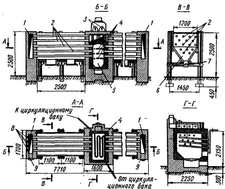
Рис. 45: Печь для подогрева сыпучих строительных материалов:
