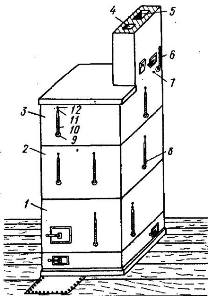
Рис. 93. Печь, оборудованная измерительными приборами для испытания: 1 — нижний пояс, 2 — средний пояс, 3 — верхний пояс, 4 — вентиляционный канал, 5 — дымовая труба, 6 — угловой термометр, 7 — место установки тягомера, 8 — ртутный термометр, 9 — гипсовое вяжущее, 10 — термометр, 11 — нить, 12 — гвоздь
