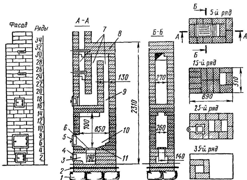
Рис. 7. Печь О-2:
