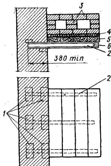
Рис. 78. Основание под печь верхнего этажа в каменном здании: 1 — металлические подкладки, 2 — швеллеры, 3 — шланцы, 4 — войлок, 5 — доски, 6 — болт
