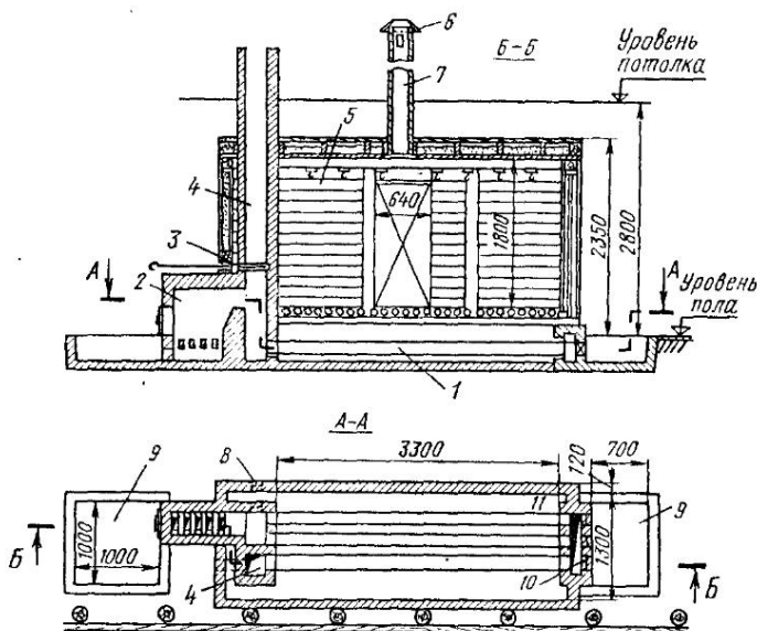
Рис. 46. Печь дезинфекционной камеры:
