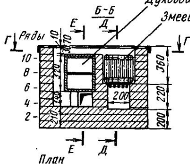
Духовой шкаф
