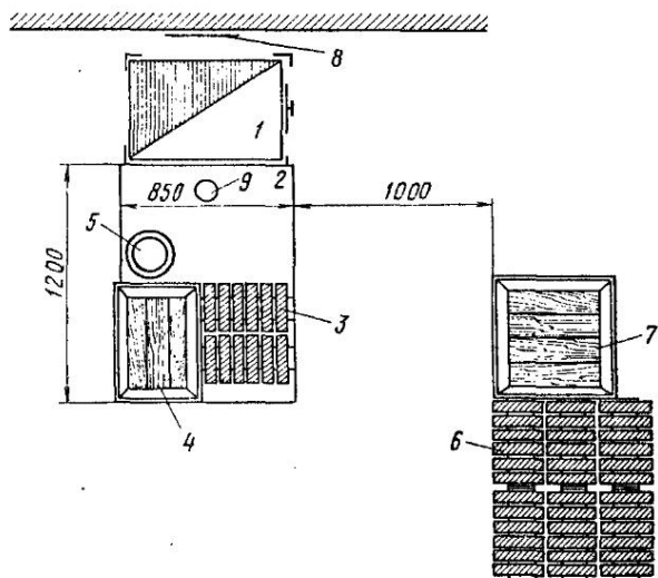
Рис. 106. Схема организации рабочего места при кладке малогабаритной печи в каркасе:
