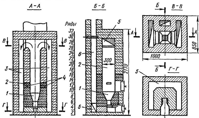
Рис. 18. Печь Теплотехнического института:
