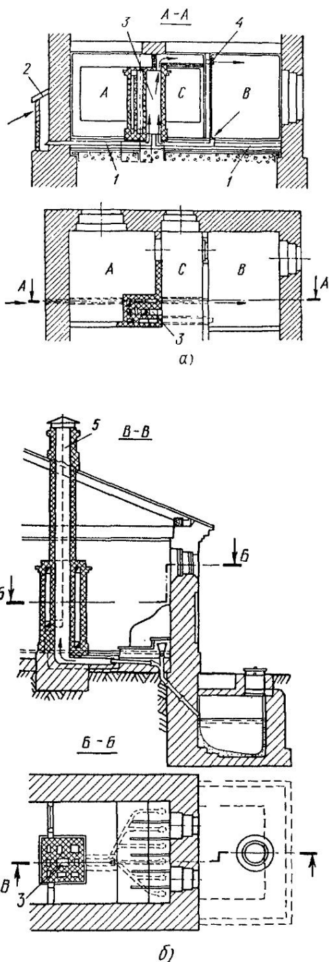
Рис 48. Отопительно-вентиляционные печи, работающие а — на приток б — на вытяжку; 1 — каналы для подвода воздуха 2 — воздухозаборная шахта 3 — воздушная камера (ВК). 4 — клапан хлопнушка, 5 — вытяжная труба; А В С — помещения
