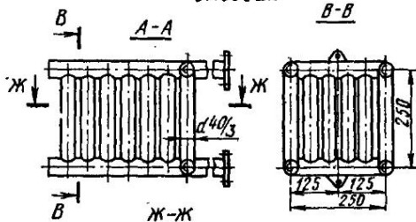
Змеевик
