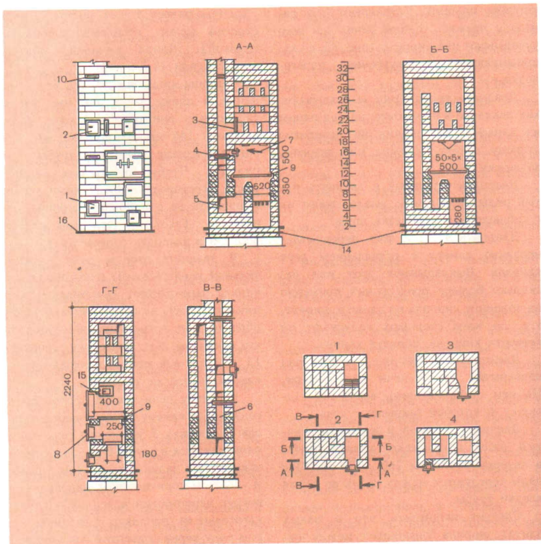
Рис. 89. Отопительно-варочная печь обычная и с тепловым шкафом:
