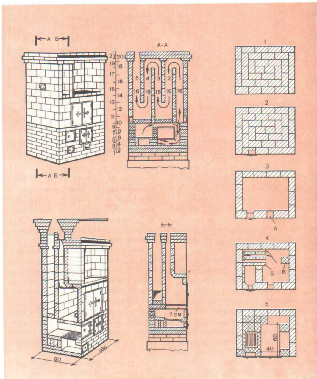
Рис. 95. Печь типа «шведка» конструкции К. Я. Буслаева
