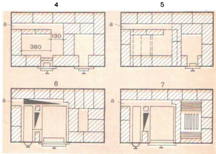
Рис. 63. Варианты отвода дымовых газов с торцевой стороны плиты:
