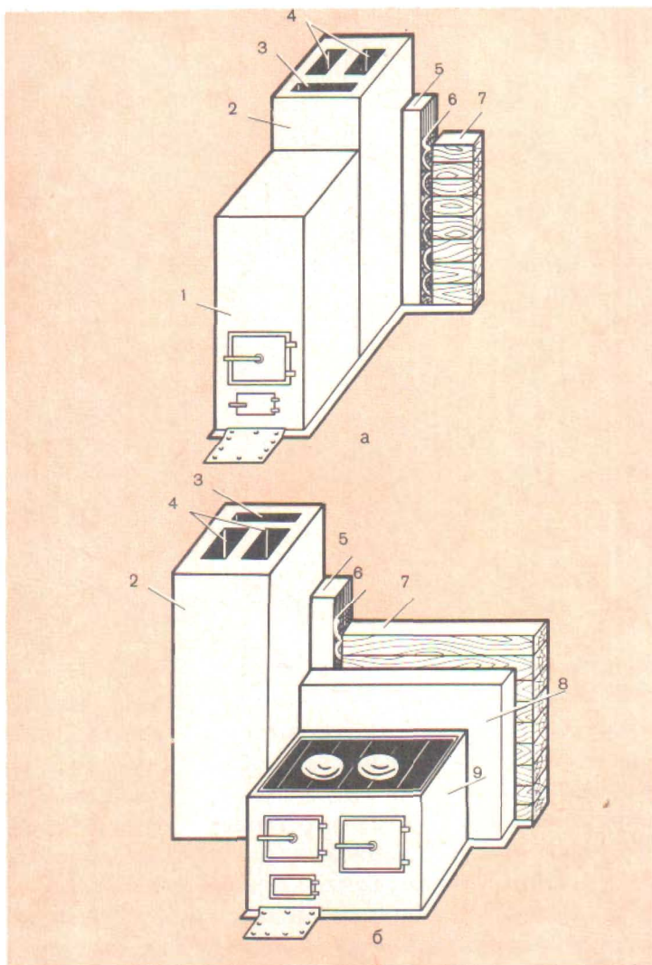
Рис. 119. Коренные трубы с подключенными печами:
