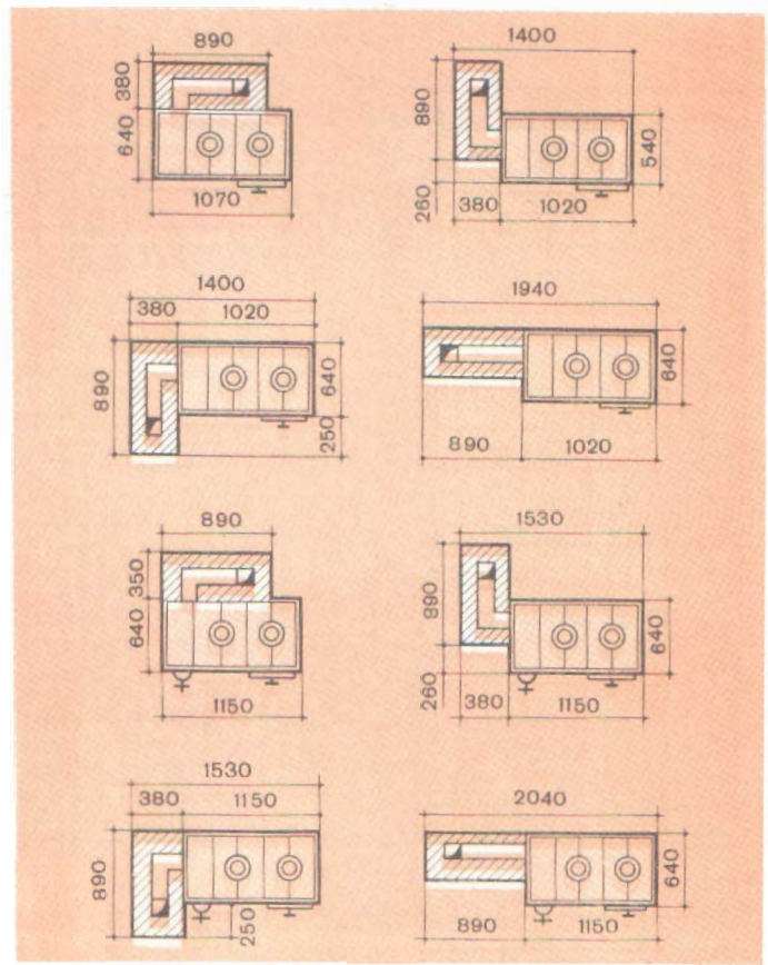
Рис. 64. Схемы присоединения плиты к отопительным щиткам
