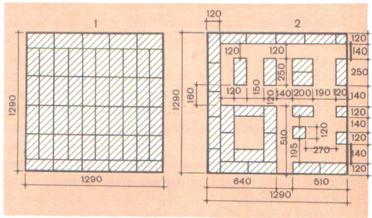
Рис. 85. «Теплушка-2» размером 1290 × 1290 мм. Печь кладет- ся, как предыдущая. Детали те же. Показаны ряды 1-й и 2-й
