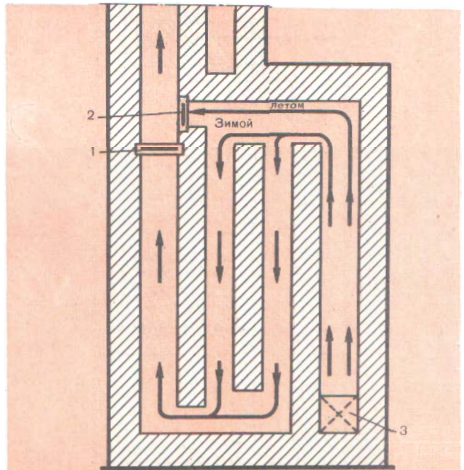
Рис. 67. Отопительный щиток с двумя хо- дами: зимним и летним: 1 — зимняя задвижка; 2 — летняя задвижка; 3 — место подключения плиты
