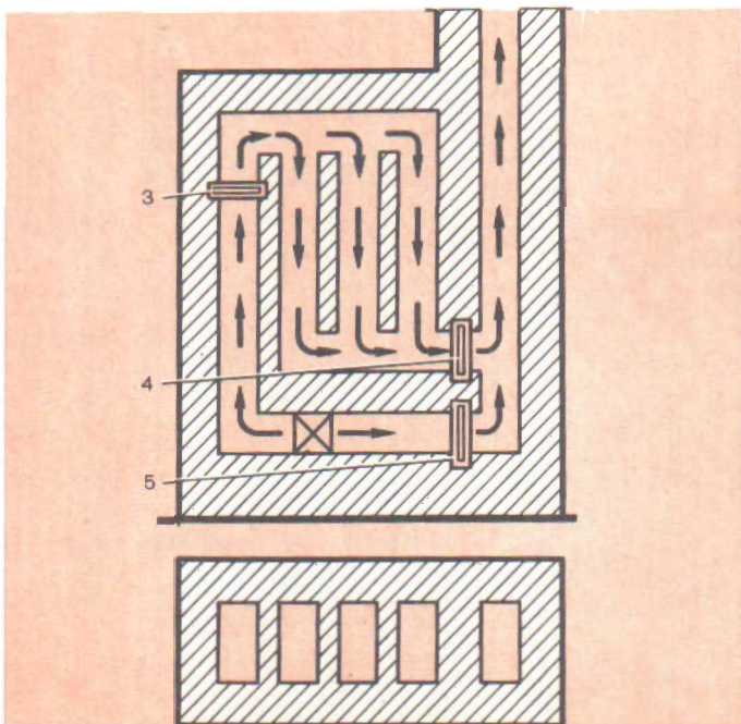
Рис. 69. Отопительный щиток толстостенный: 1 — места присоединения кухонной плиты; 2 — чистка; 3 — гидроизоляция; 4 — самоварник; 5 — вентиляционная решетка с клапаном
