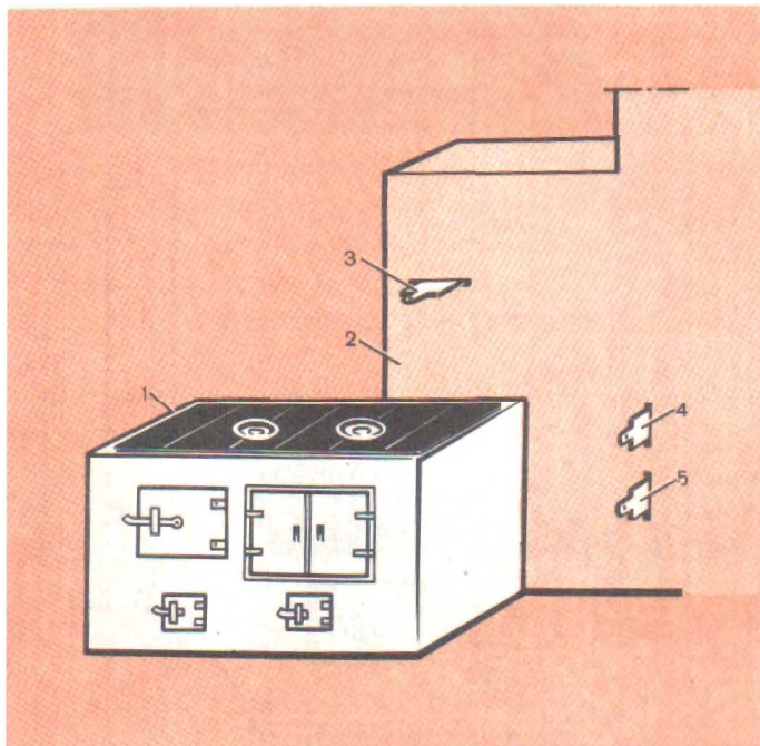
Рис. 68. Разрез щитка с задвижками, расположенными сверху и внизу: 1 — чугунный настил (плита) с двумя конфорками; 2 — щиток; 3 — задвижка для перекрытия каналов; 4, 5 — задвижка для регулировки движения газов в летнее и зимнее время
