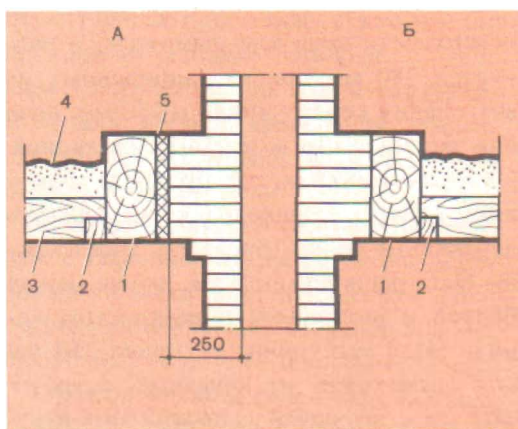
Рис. 130. Изоляция концов балок в печной кладке около каналов
