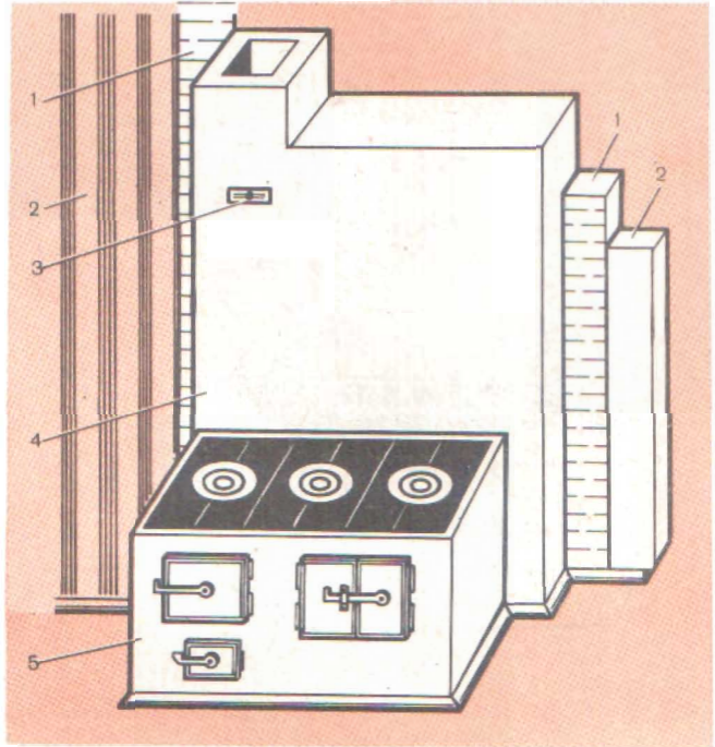
Рис. 66. Кухонная плита с постоянно на- грываемым отопительным щитком: 1 — кирпичная разделка; 2 — перегородки (стенки); 3 — дымовая задвижка; 4 — щиток; 5 — плита
